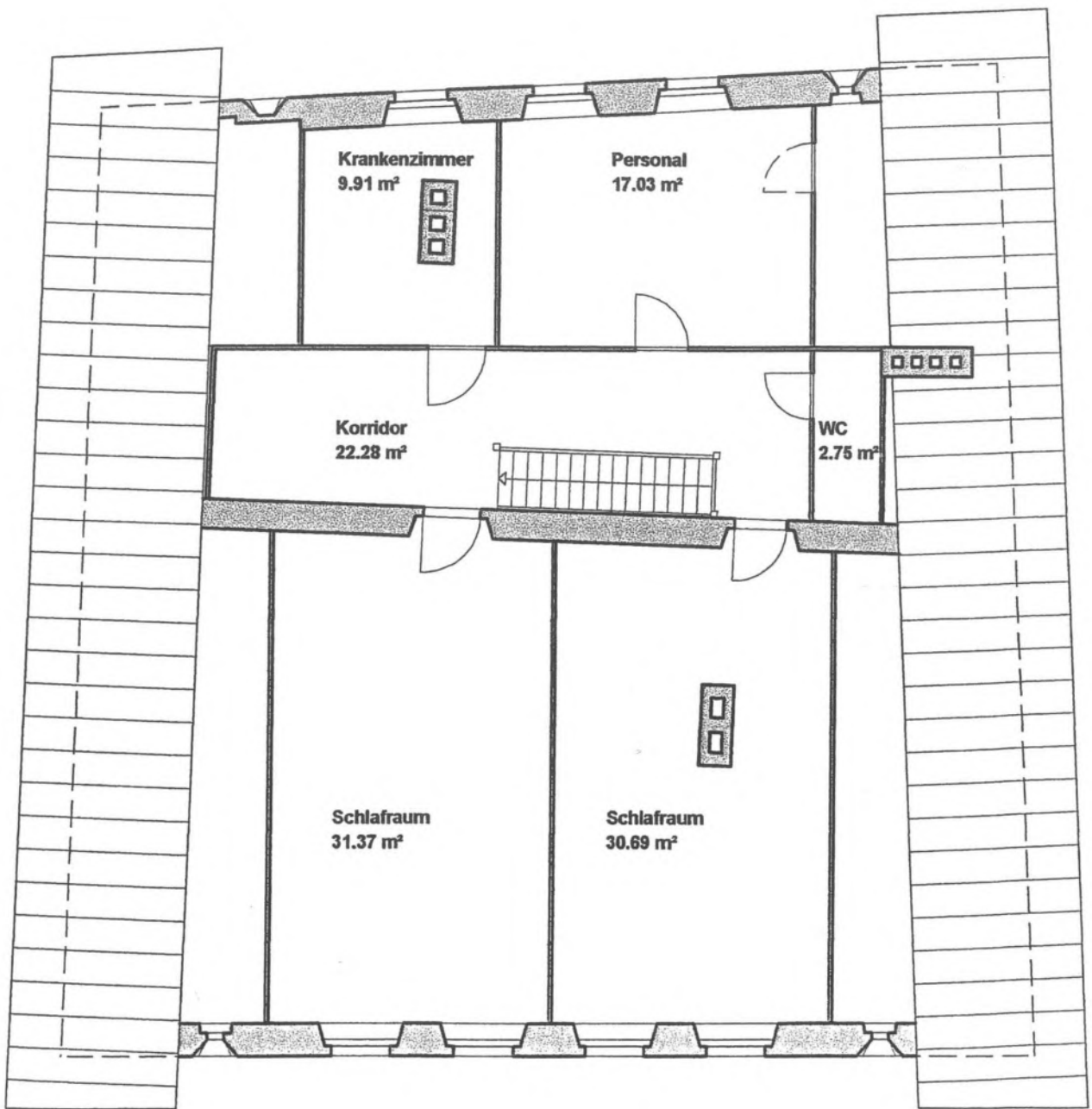
Ferienkolonie Valbella Dachgeschoss 1:100
